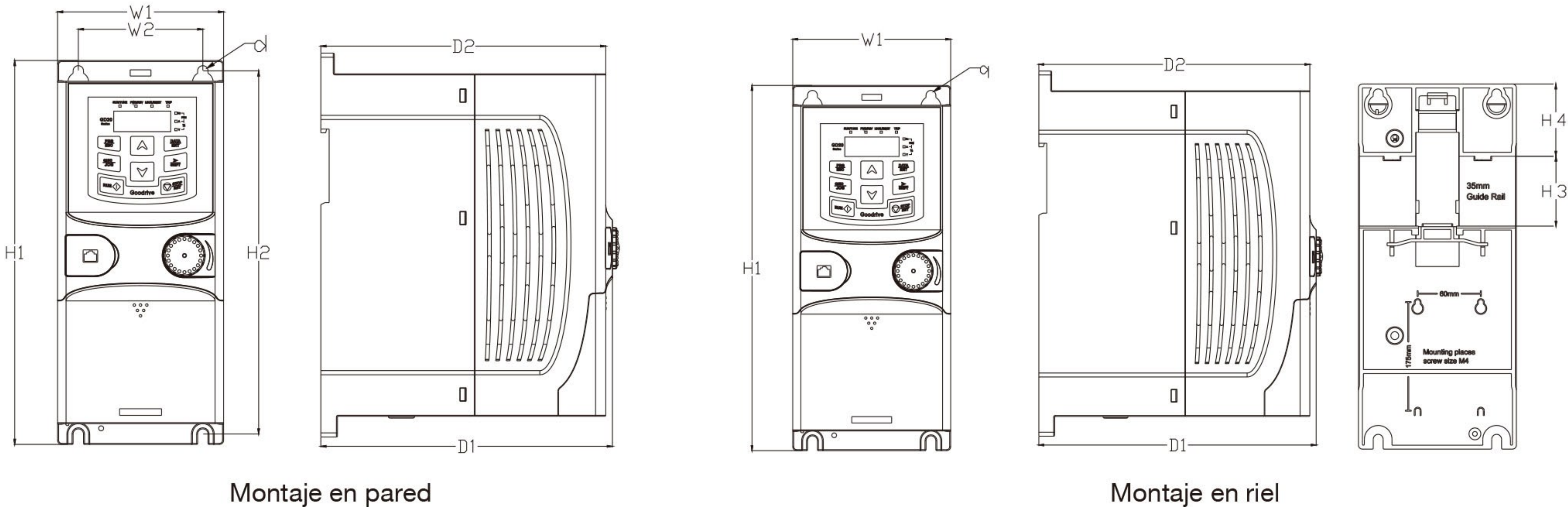
Dimensiones del montaje en pared (unidad: mm)
