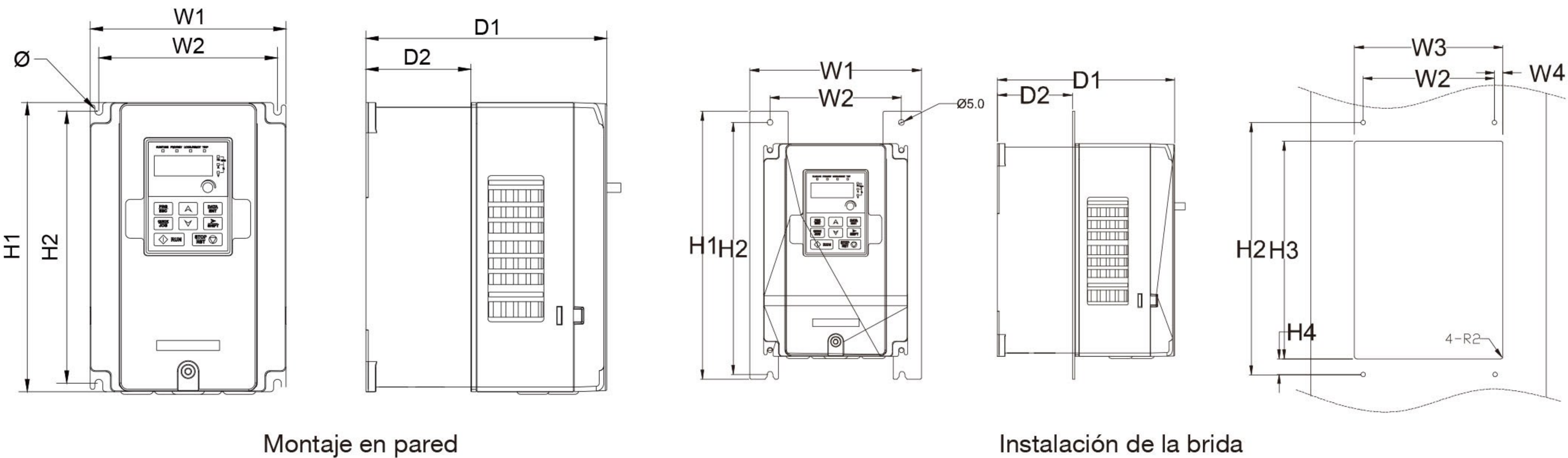
Dimensiones del montaje en pared (unidad: mm)
