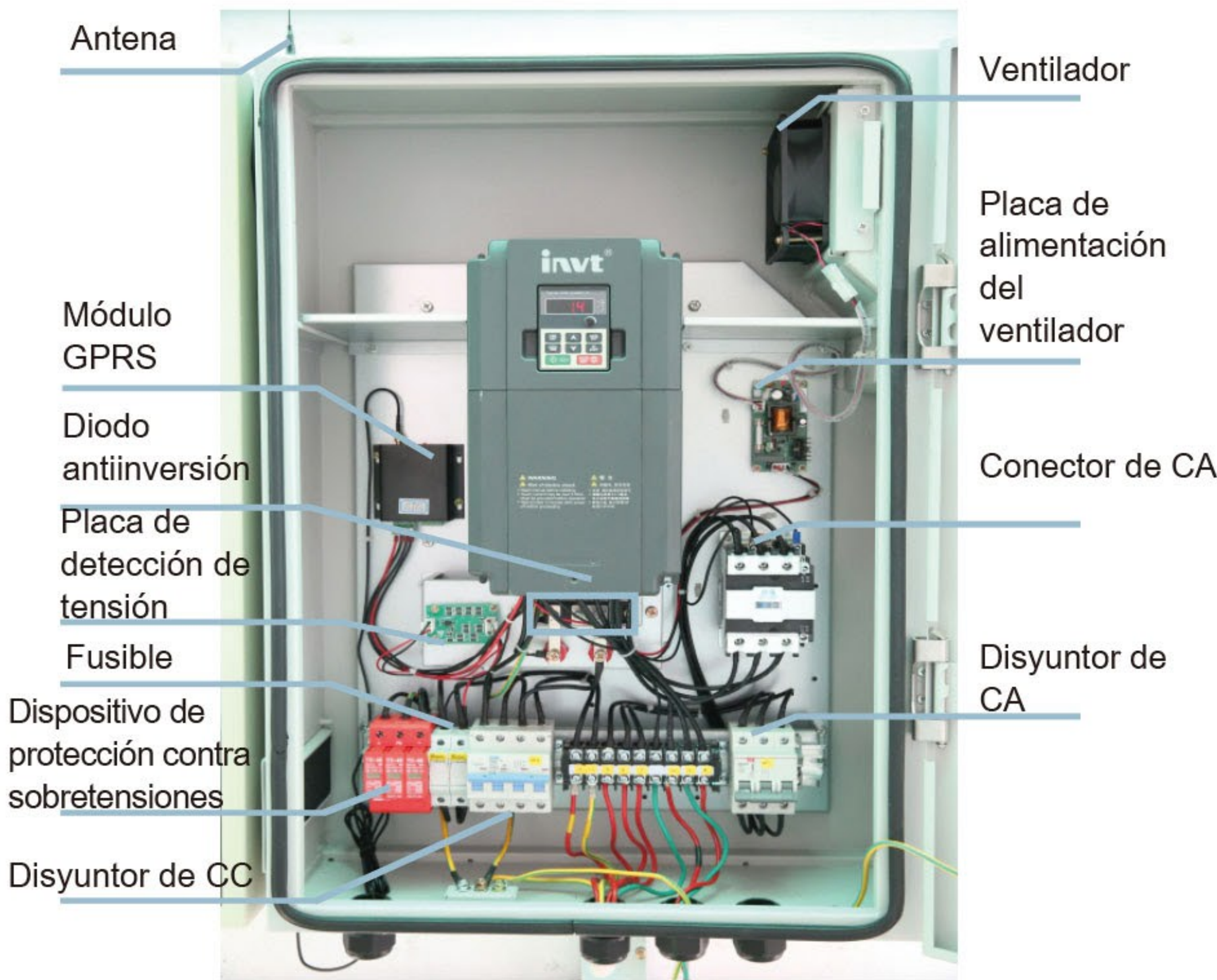
Estructura interna de GD100-015G-45-PV-AS
